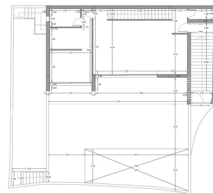
Planta Baja, escala 1:100
