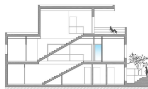
Sección A-A, escala 1:100
