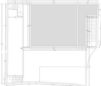
Planta Tercera, escala 1:100
