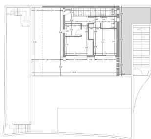
Planta Segunda, escala 1:100
